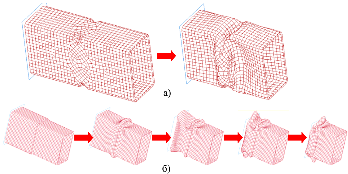
Рис. 3.33. Моделирование деформации крашбоксов: а – с заломами на ребрах; б – переменного сечения
