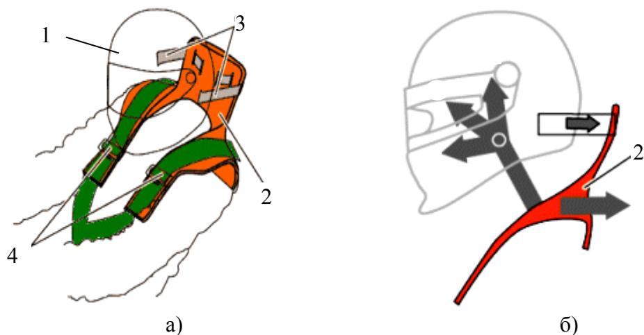
Рис. 3.16. Система удержания головы HANS (а) и схема перераспределения сил, действующих на голову в шлеме на воротник системы (б): 1 – шлем; 2 – воротник; 3 – ремни, соединяющие шлем и воротник; 4 – грудные ленты шеститочечных ремней безопасности
