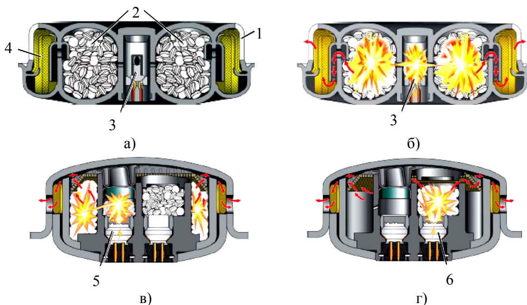
Рис. 3.10. Газогенератор водительской подушки безопасности: а – одноступенчатый газогенератор; б – активирован одноступенчатый газогенератор; в – активирована первая ступень двухступенчатого газогенератора; г – активирована вторая ступень двухступенчатого газогенератора; 1 – корпус; 2 – заряд; 3 – активатор (запал) пороховой; 4 – сетка для фильтрации крупных частиц заряда; 5 – активатор первой ступени; 6 – активатор второй ступени
