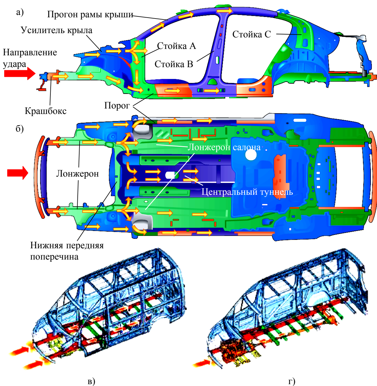
Рис. 3.24. Распределение энергии фронтального удара (показано стрелками) по силовой структуре несущего кузова и раме автомобиля: а – вид сбоку ( VolkswagenPassat B6 ); б – вид снизу ( VolkswagenPassat B6 ); в – по раме Volkswagen Crafter ; г – через силовой агрегат на раму Volkswagen Crafter
