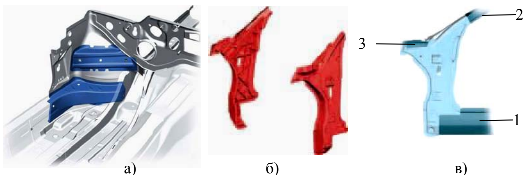
Рис. 3.27. Распределение нагрузки на стойку А силового каркаса салона Audi : а – распределитель нагрузки лонжерон (усилитель крыла) – стойка А; б – левая и правая стойки; в – силовое взаимодействие стойки А с другими элементами: 1 – порог; 2 – прогон рамы крыши; 3 – усилитель крыла
