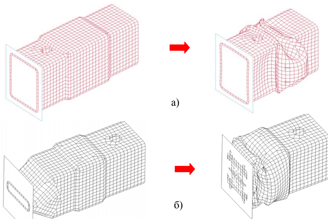
Рис. 3.32. Моделирование деформации крашбоксов: а – Volkswagen Golf V ; б – Volkswagen Tiguan
