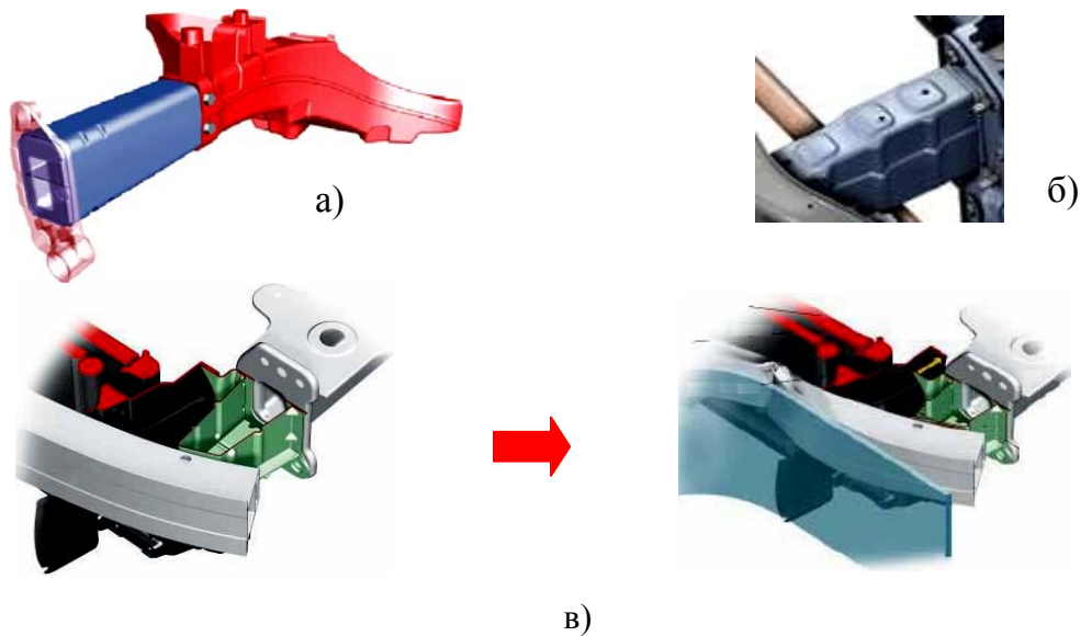
Рис. 3.34. Крашбоксы с заломами Audi A2 (а), с готовыми складками Mercedes ML (б) и Audi A3 (б)
