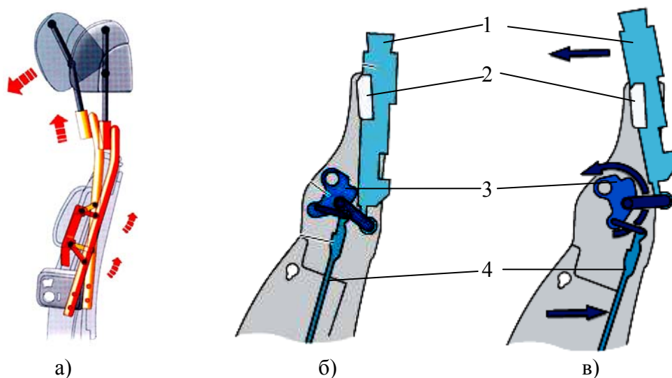
Рис. 3.15. Активные подголовники Peugeot 307 (а) и Audi А6 в исходном (б) и активированном (в) состоянии:
