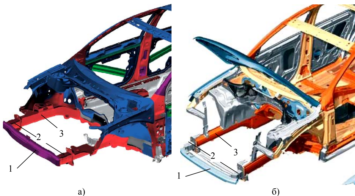
а) б) Рис. 3.25. Силовая структура передней части автомобилей Volkswagen Golf (а) и Audi Q7 (б): 1 – поперечина; 2 – крашбокс; 3 – лонжерон
