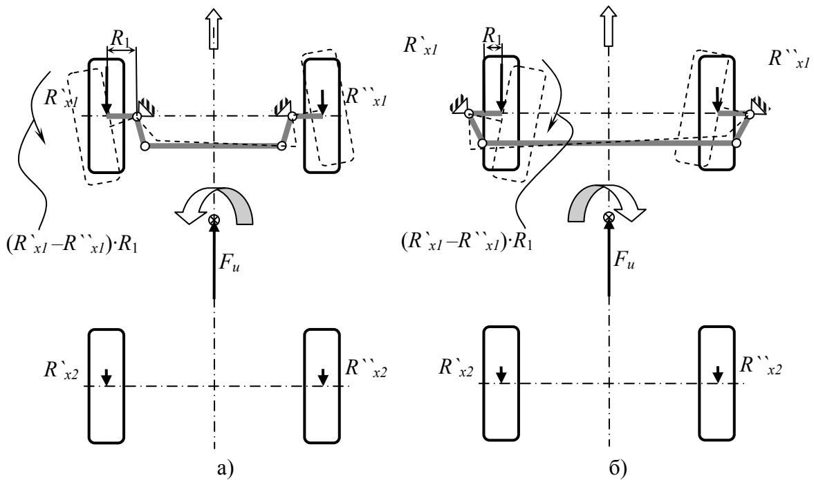
Рис. 1.7. Влияние положительного (а) и отрицательного (б) плеча обкатки r_s = R_1 / \cos \sigma (см. рис. 1.6) на устойчивость автомобиля при торможении:
