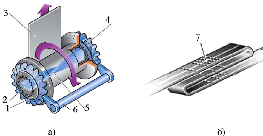
Рис. 3.6. Ограничители усилия на ремне безопасности: торсионный (а) и S-образный (б); 1 – ступица катушки; 2 – торсионный вал (уже скрученный); 3 – ремень безопасности; 4 – зубчатое колесо; 5 – катушка ремня; 6 – стопор; 7 – сквозная прошивка ремня
