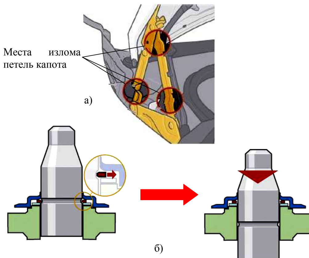
Рис. 3.39. Меры по снижению травм пешеходу ( Volkswagen Golf 2009 г.): а – излом петель капота; б – утапливающийся вал привода стеклоочистителя
