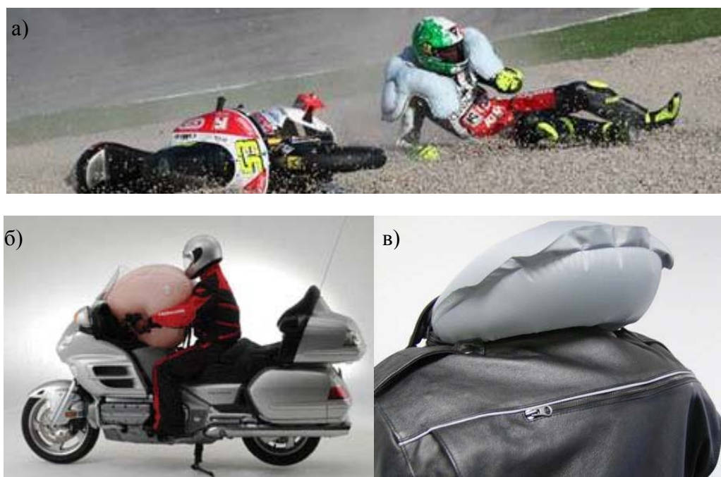
Рис. 3.9. Подушки безопасности современных мотоциклов: а – встроенная в экипировку спортсмена класса SuperBike (экспериментальная); б – встроенная в мотоцикл Honda ; в – встроенная в воротник куртки
