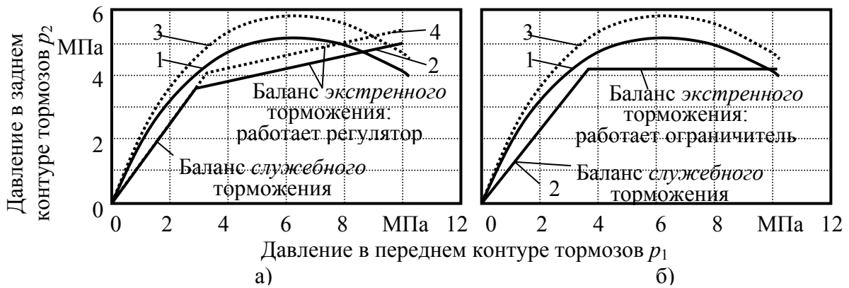
Рис. 1.4. Диаграмма работы регулятора (а) и ограничителя (б) давления в заднем контуре тормозов:
