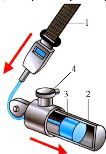
Рис. 3.5. Замочный натяжитель ремня безопасности: 1 – ремень; 2 – цилиндр; 3 – поршень; 4 – пиропатрон
