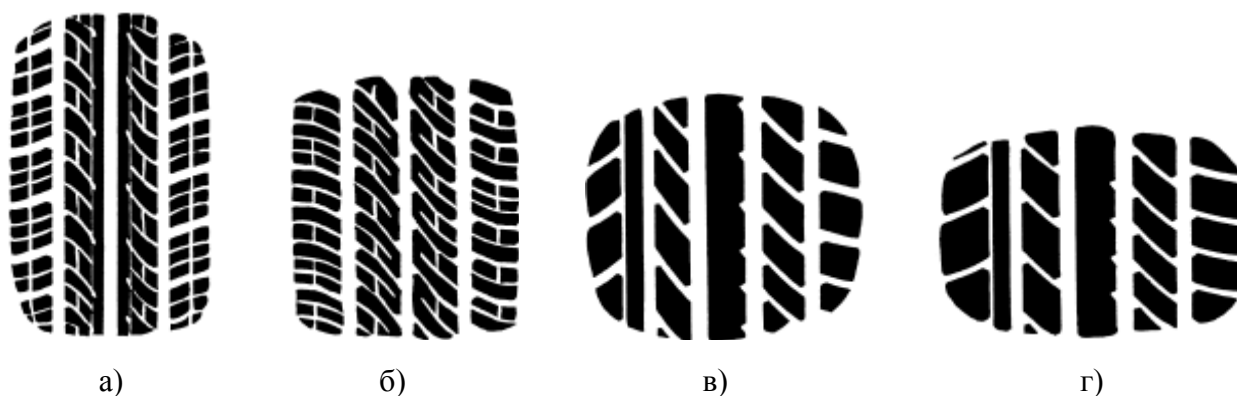
Рис. 1.2. Влияние размеров шин на форму пятна контакта (номинальный радиус шин одинаковый r_0 = 0.317 м):
