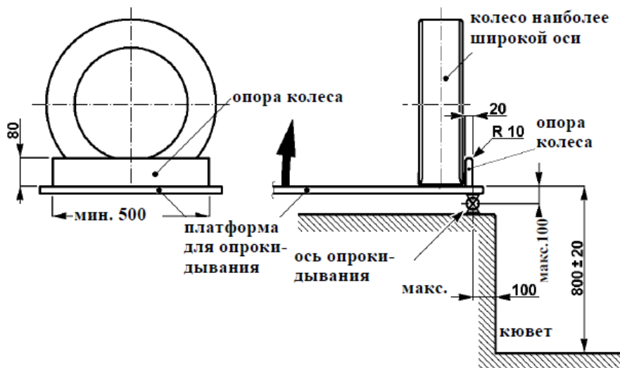
Рис. 2.13. Стенд для испытания автобуса на опрокидывание по правилу ЕЭК ООН №66
