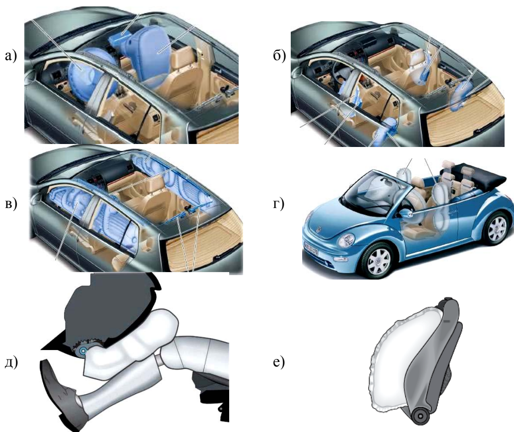
Рис. 3.8. Подушки безопасности современных автомобилей (на примере Volkswagen ): а – фронтальные (водителя и переднего пассажира); б – боковые; в – головные (шторки); г – комбинированные (боковые и головные); д – коленная; е – боковая водительская
