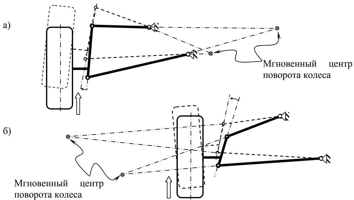
Рис. 1.10. Центр поворота колеса на двойных поперечных рычагах подвески: а, б – ориентация рычагов, соответственно обеспечивающая и не обеспечивающая перпендикулярность шины к дороге на ходе сжатия подвески
