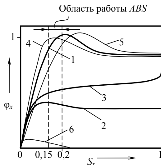
Рис. 1.3. Зависимость коэффициента продольного сцепления шины с дорогой \varphi_x от коэффициента скольжения S_x в их контакте ( \varphi – S (фи–эс) диаграмма): 1 – на сухой чистой твердой дороге; 2 – на льду или укатанном снегу; 3 – на твердой дороге, покрытой песком или рыхлым снегом; 4, 5 – при избыточном и недостаточном давлении в шинах соответственно; 6 – при аквапланировании
