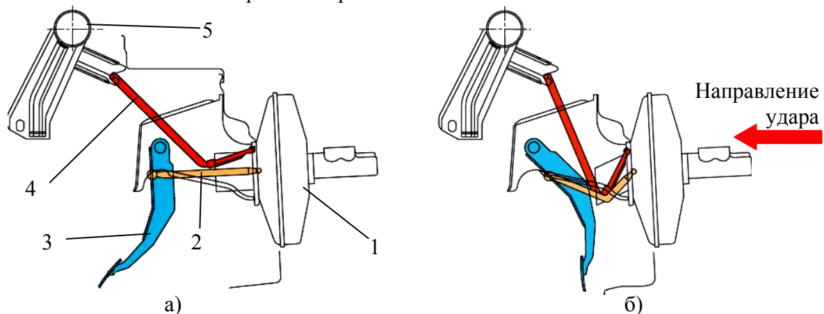
Рис. 3.22. Педальный узел Volkswagen Beetle до столкновения (а) и после (б): 1 – главный тормозной цилиндр с усилителем; 2 – шток; 3 – тормозная педаль; 4 – кронштейн; 5 – поперечина каркаса безопасности автомобиля
