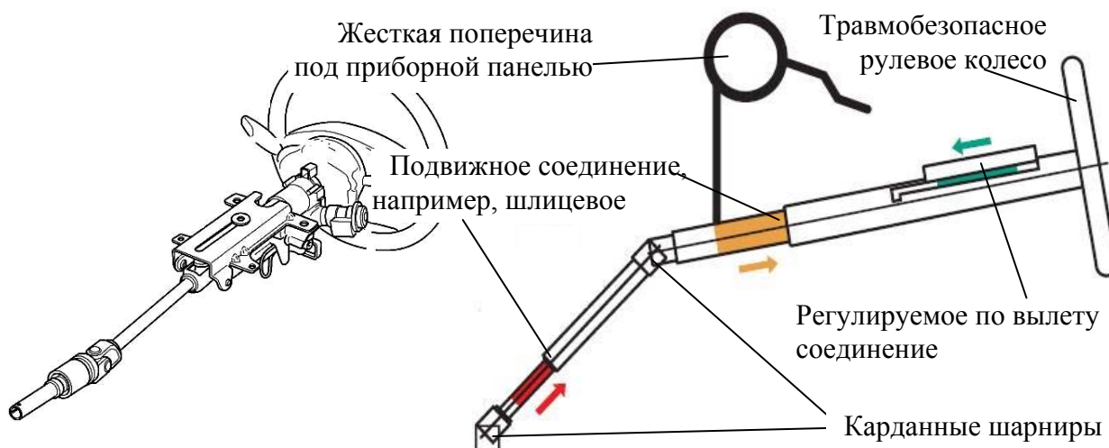
Рис. 3.18. Травмобезопасная рулевая колонка автомобиля с несущим кузовом
