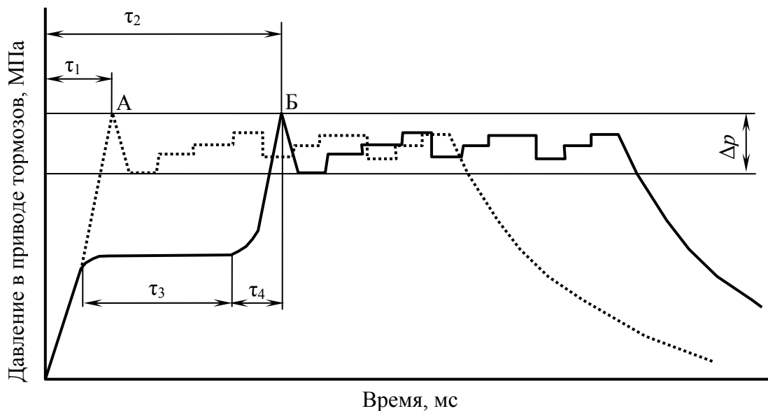
Рис. 1.5. Диаграмма работы усилителя экстренного торможения BA :
