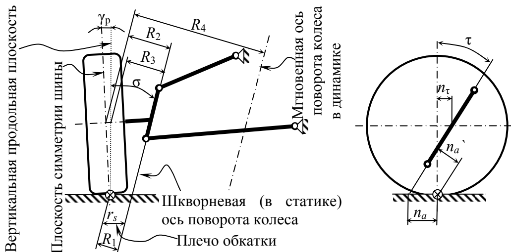
Рис. 1.6. Параметры установки управляемых колес
