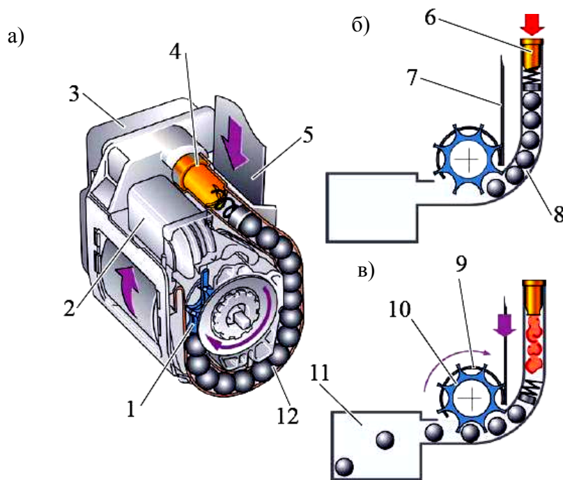
Рис. 3.3. Шариковый натяжитель ремня безопасности (а) и схема его работы в начальной (б) и промежуточной фазе (в):
